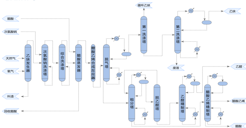
醋酸乙烯生产工艺流程图（天然气法）
