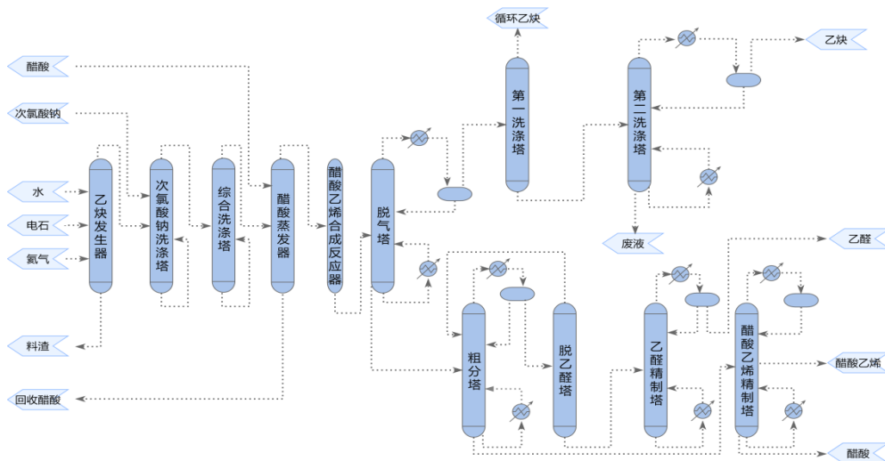
醋酸乙烯生产工艺流程图（电石法）
