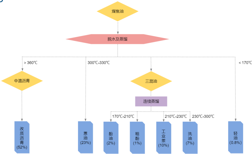
煤焦油深加工工艺流程图
