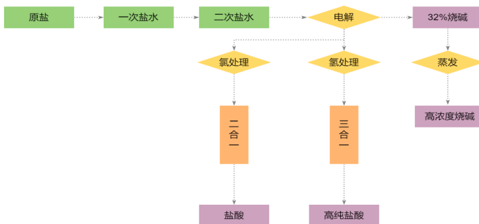
氯碱生产工艺流程图
