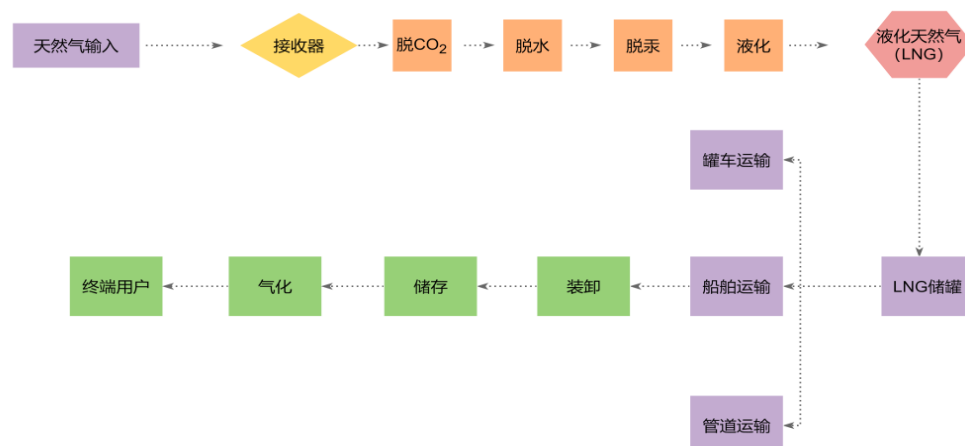
液化天然气生产工艺流程图（液化制冷）
