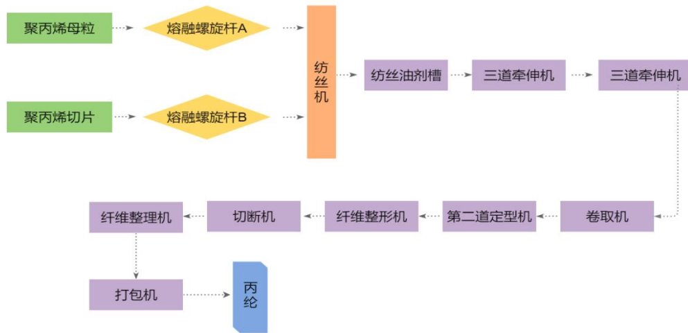
丙纶生产工艺流程图
